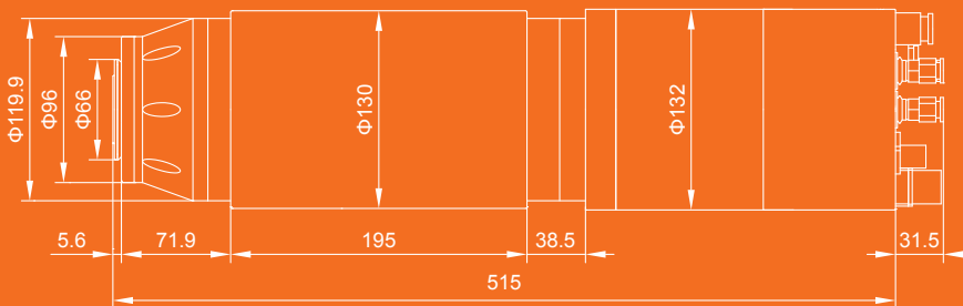
尺寸图(mm)
